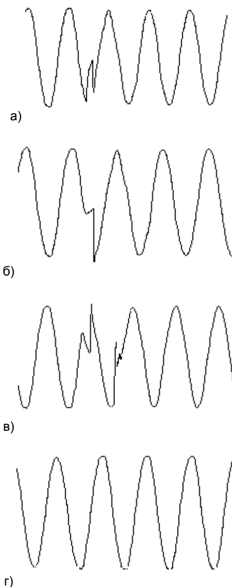
Рис. 13. Осциллограммы переключения «сеть-батарея» (а, б, в) и «батарея-сеть» (г) для ИБП, взаимодействующего с сетью
