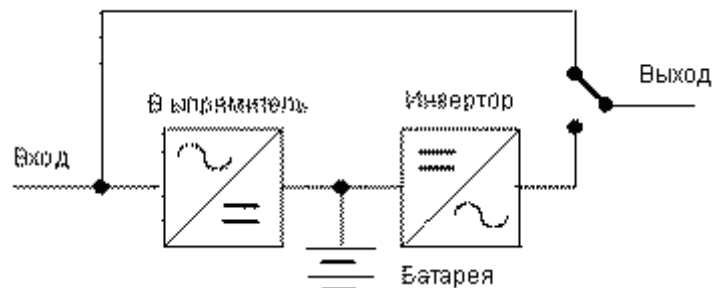
Рис. 5. ИБП с переключением
